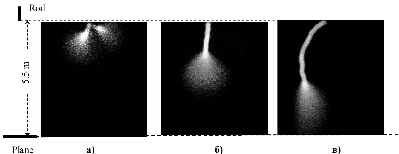
Рис.7. Камера К008: типичные картины развития положительного лидера при импульсе напряжения +130/7500\text{мкс} , U=2\text{МВ} (позитивное изображение, длительность кадра 6мкс). Снимки относятся к разным разрядам: а) - начало, б) - середина, в) - конец лидерной стадии.
