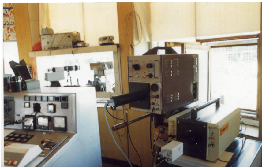
Рис.2. Общий вид комплекса электронно-оптической аппаратуры.
